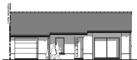
FACADE AVANT
